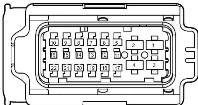
DR21 左后门线束接底板线束连接器
