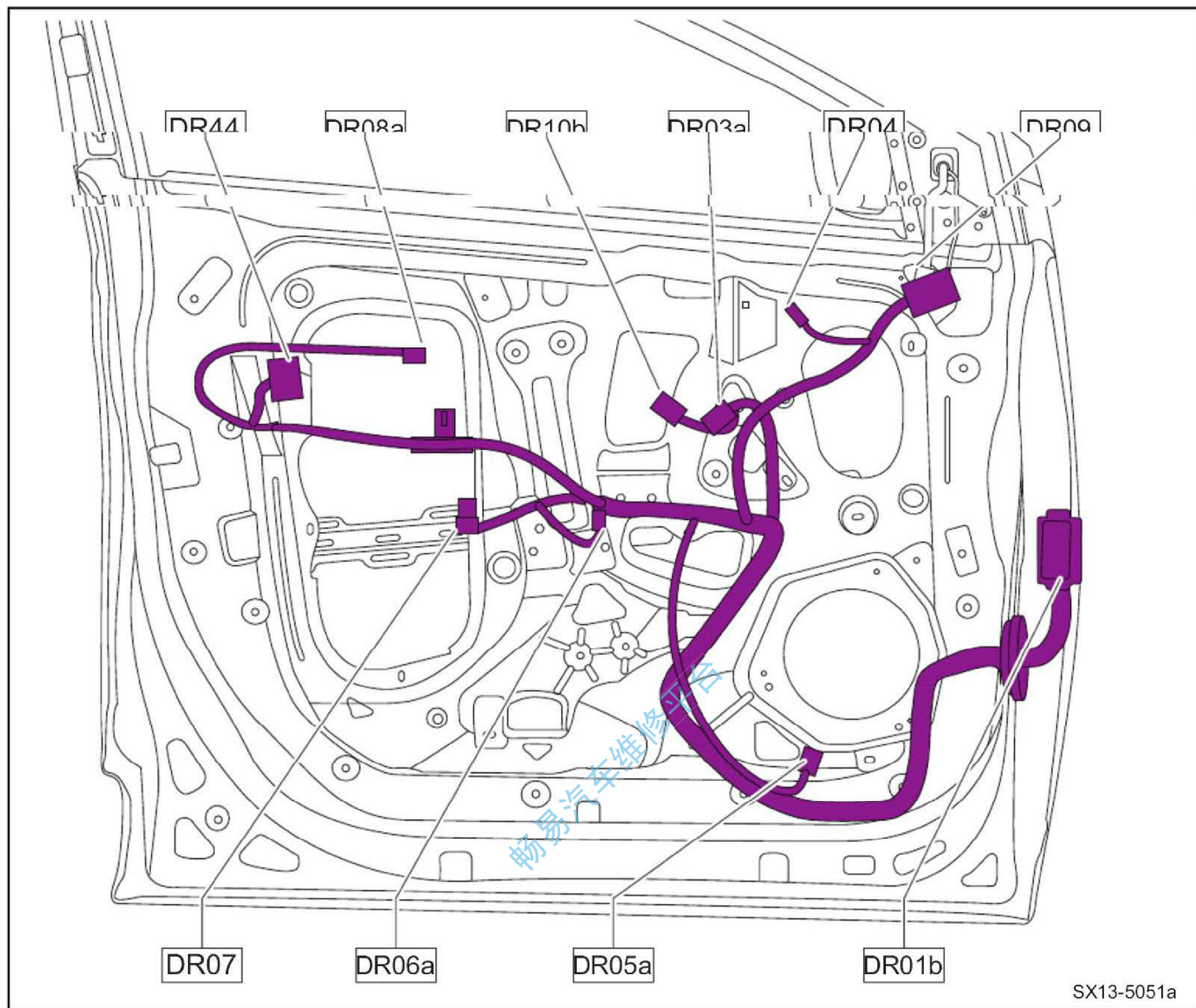
左前门线束布置图
