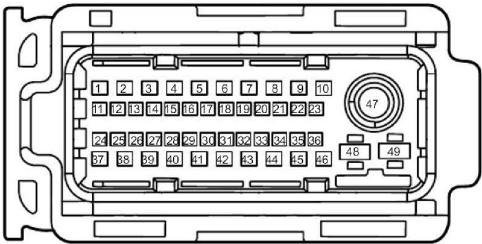
DR04 驾驶员侧门玻璃升降器开关线束连接器
