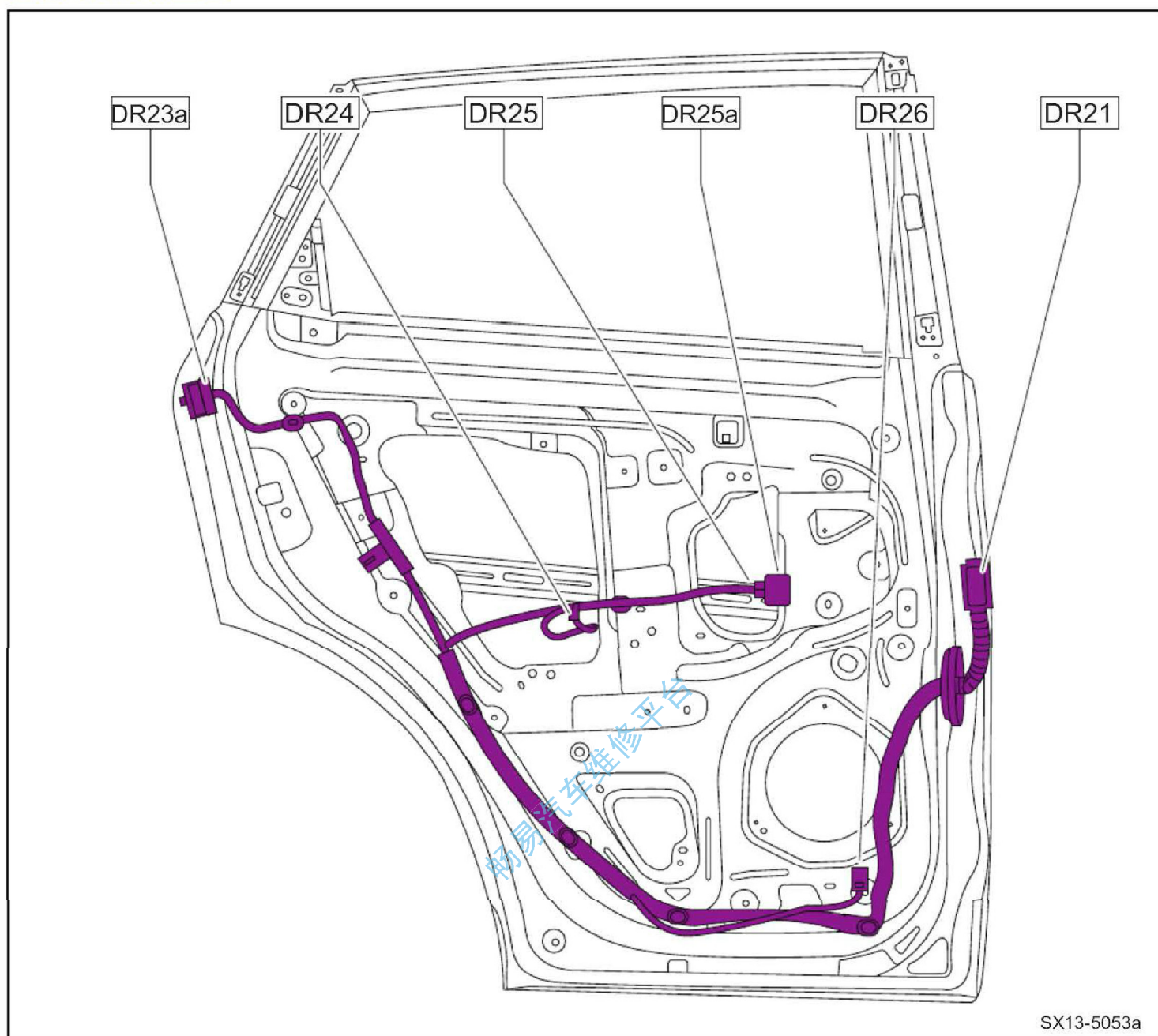
左后门线束布置图
