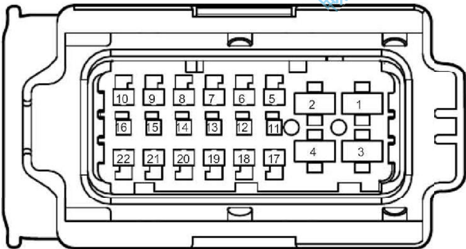
DR31 右后门线束接底板线束连接器
