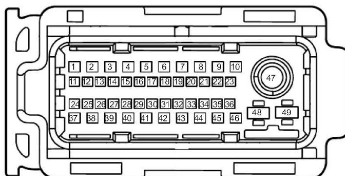
DR11b 前乘员门线束接底板线束连接器
