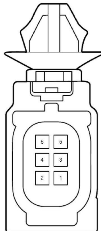
DR20b 前乘员侧门把手传感器线束连接器
