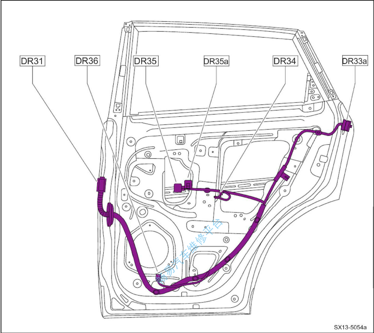
右后门线束布置图
